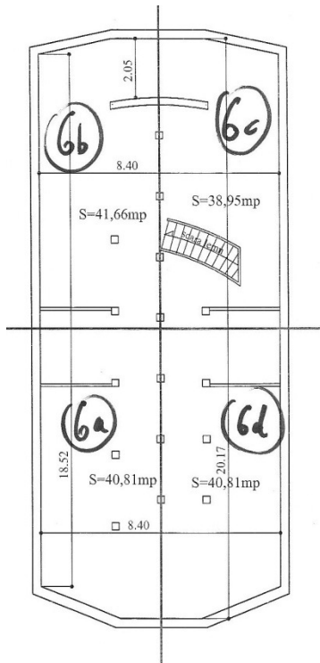
PLAN MANSARDA; Sc. 1:100 -CORP A-
