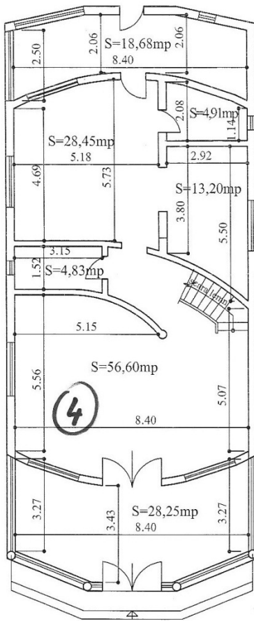
PLAN PARTER; Sc. 1:100 -CORP A-
